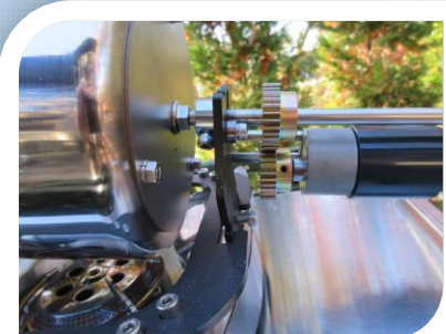
焙煎機をセット後部ギアを上下にセット。
